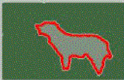
Query blobs
